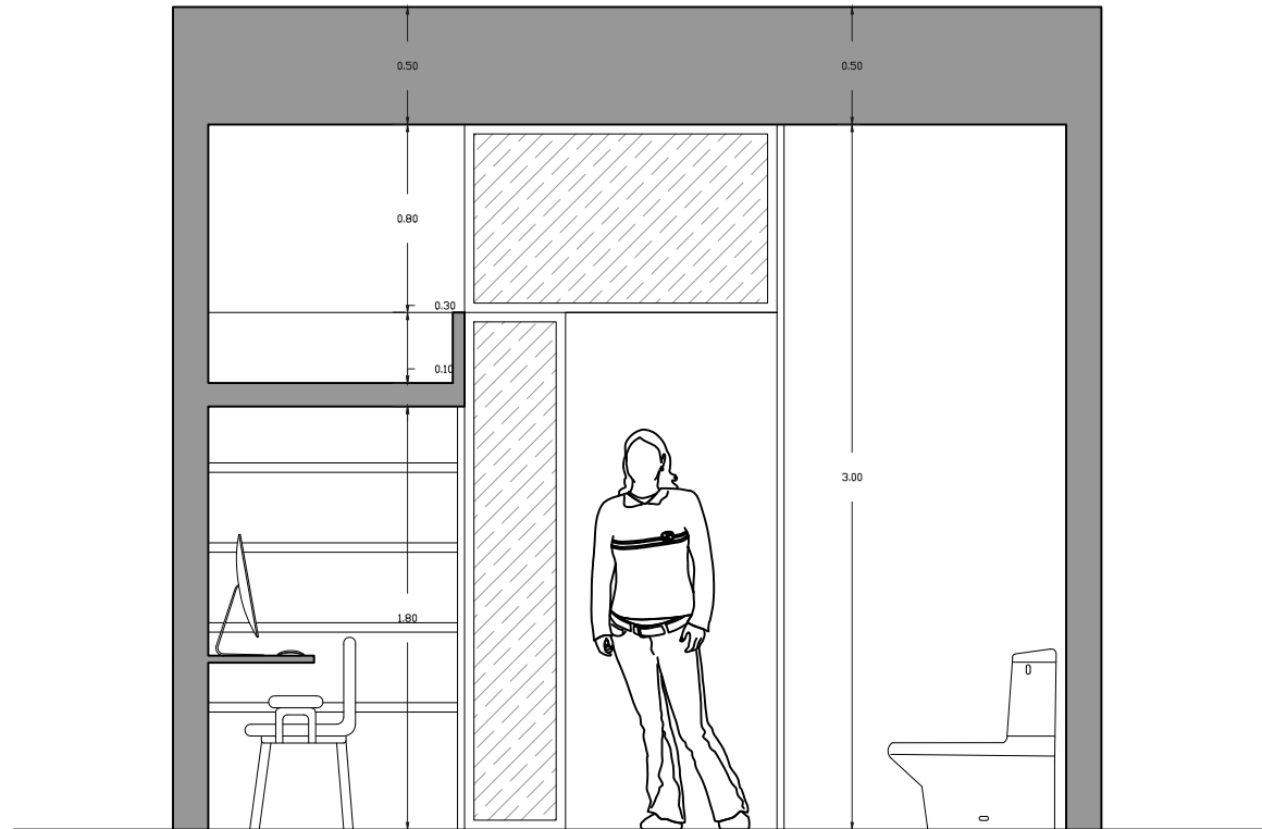
Corte vivienda individual de 12m 2 Esc 1:35
